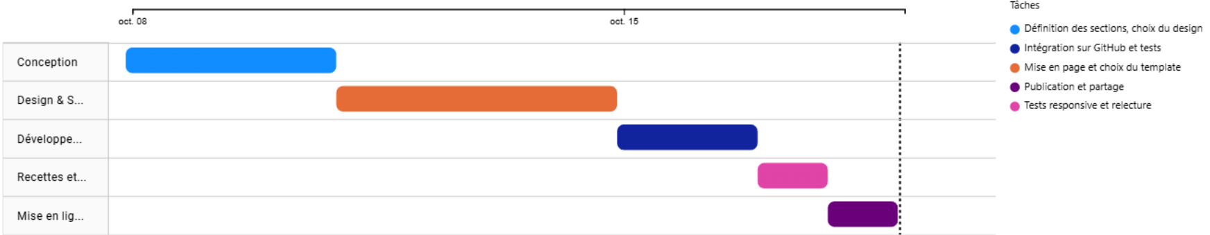
Rétroplanning (GANTT)
